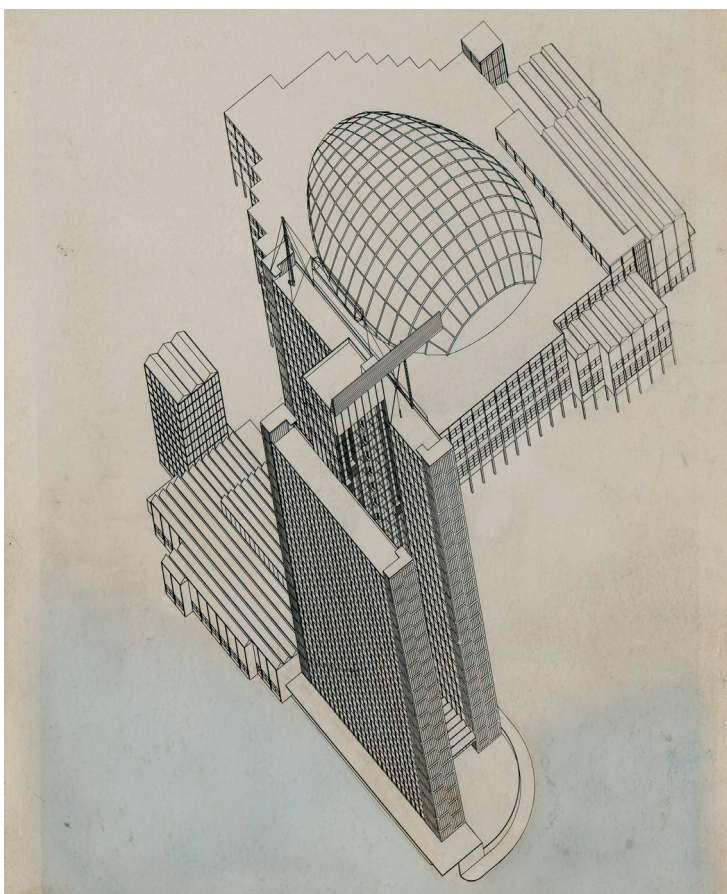
Hannes Meyer et Hans Wittwer, Projet de concours pour la Société des Nations à Genève, 1927. Axonométrie (photographie sur papier), Archives de la construction moderne (Acm) – Fonds Alberto Sartoris
